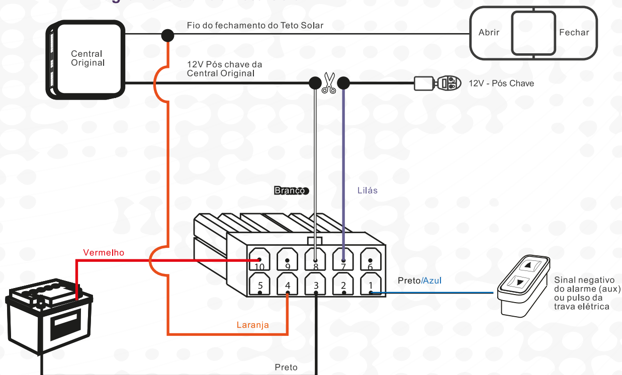
Diagrama Geral do Teto Solar
